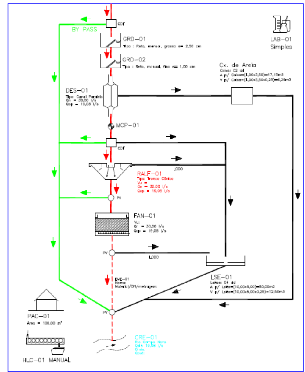
ESTAÇÃO DE TRATAMENTO DE ESGOTO DE QUEDAS DO IGUAÇU
