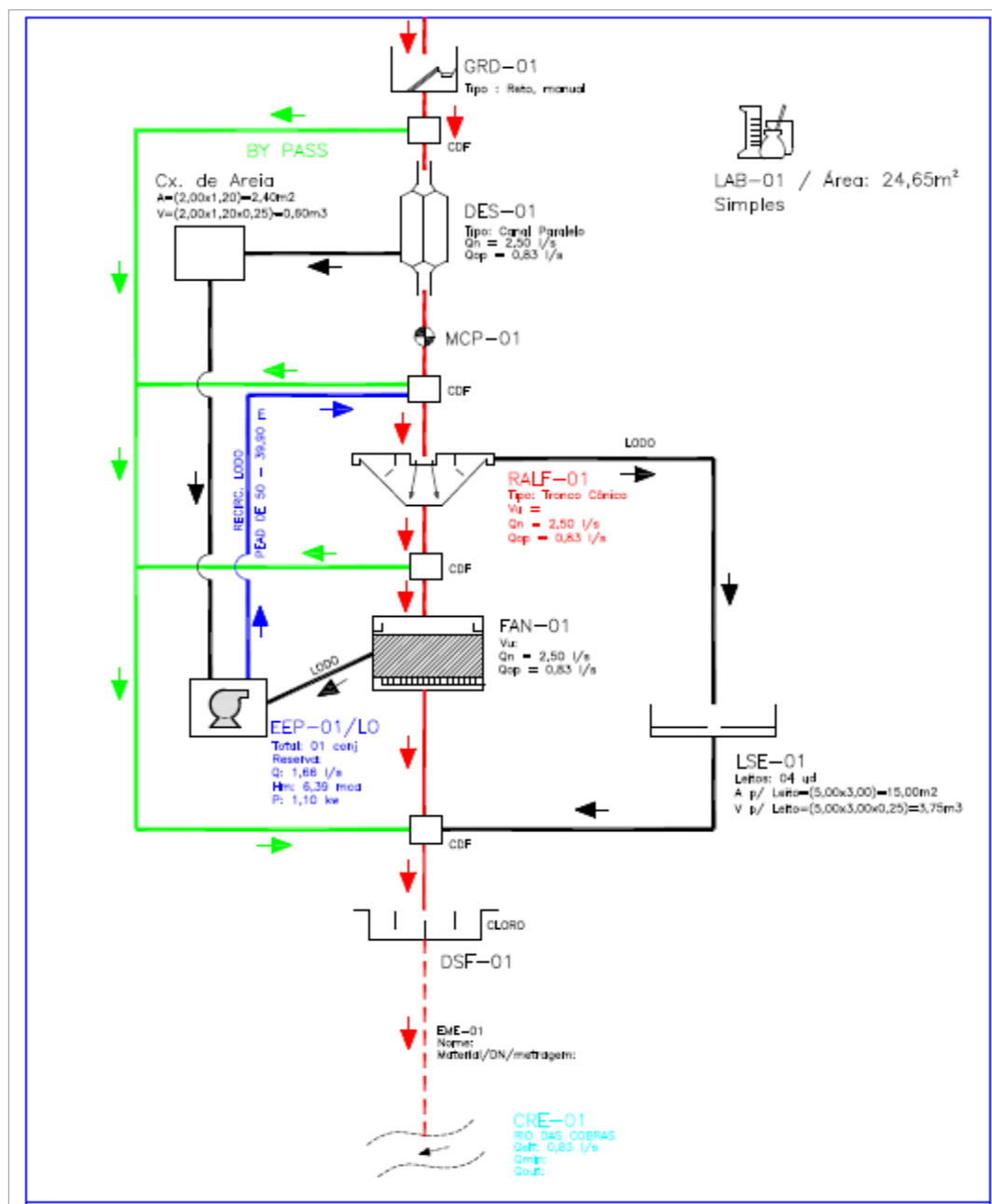
ESTAÇÃO TRATAMENTO DE ESGOTO DA VILA SALTO OSÓRIO
